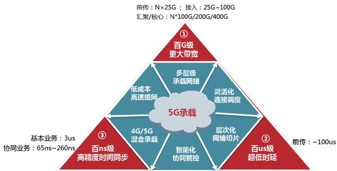
图5-1 5G承载整体需求
