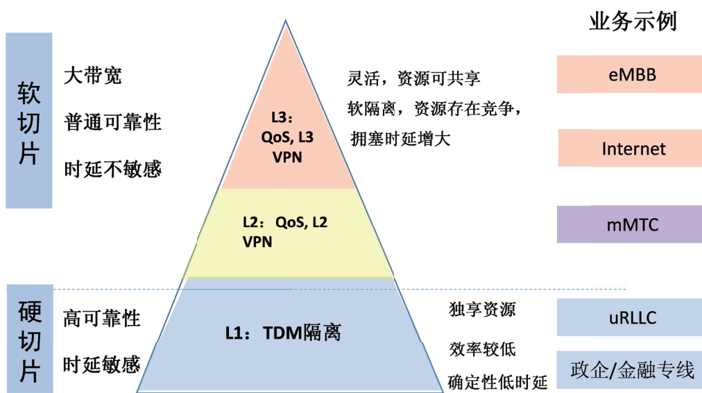
图4-3 5G承载层次化网络切片应用示意
