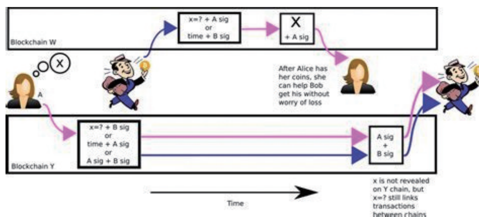
图9 基于信息锁模式的跨链资产交互
