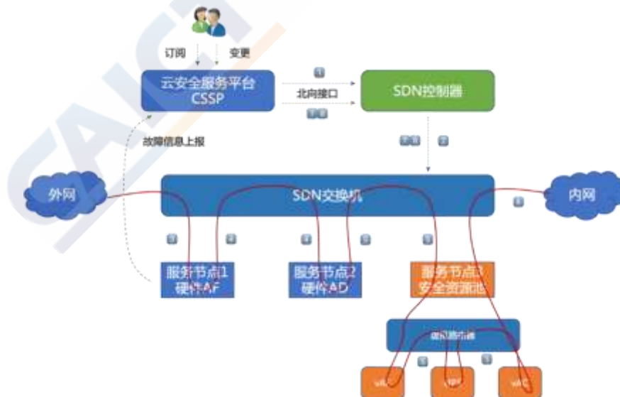
图附 23 云安全服务链技术架构
