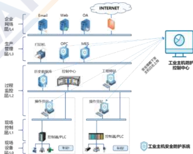
图附 10 工业主机安全防护系统部署
