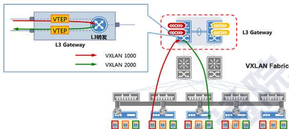
图附 21 三层网关（L3 Gateway）工作原理图
