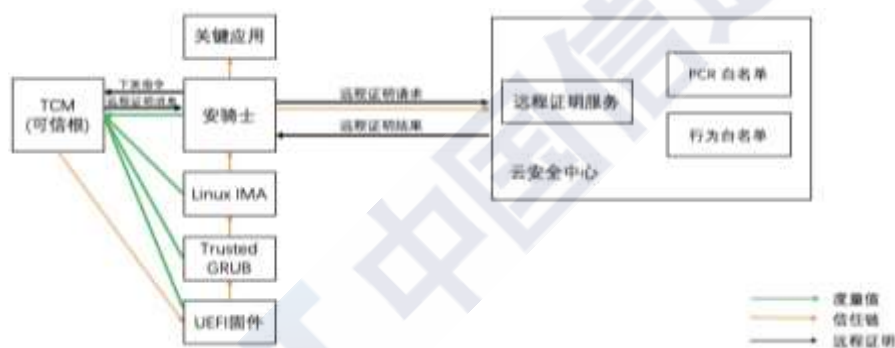
图附 27 云平台可信根实现框架图
