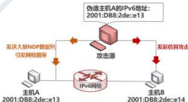
图 3.9 NDP 攻击
